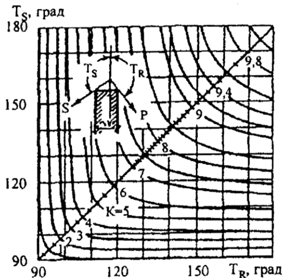
Рис. 4.13. Номограмма для определения величины K
