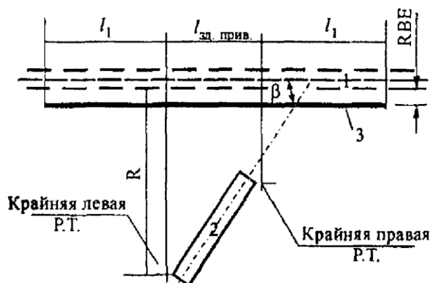
Рис. 4.4. Определение требуемой длины экрана:
