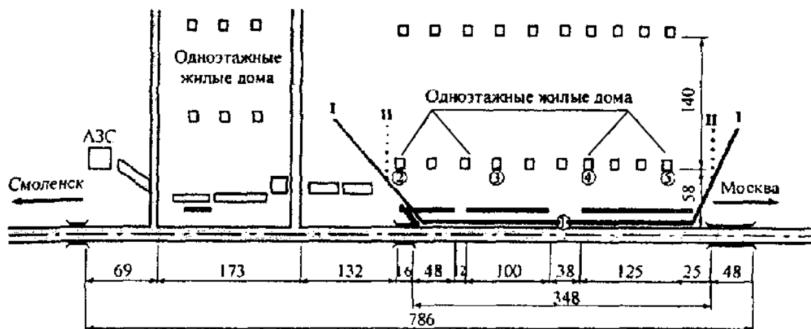
Рис. 5. Рекомендуемая схема размещения шумозащитного экрана
