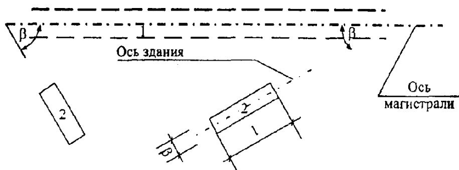
Рис. 4.5. Примеры расположения зданий под углом \beta :
