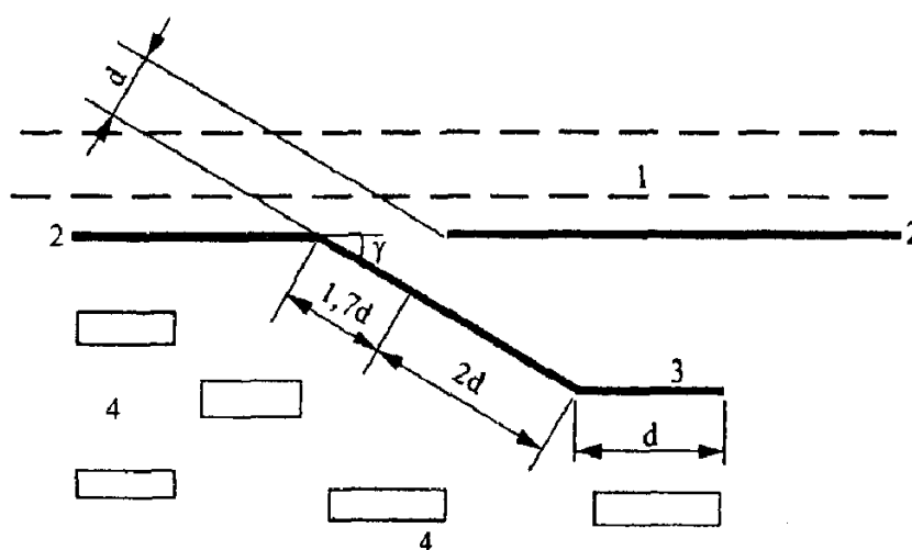
Рис. 4.10. Устройство дубль-экрана при организации прохода (проезда) на территорию за основным экраном:
