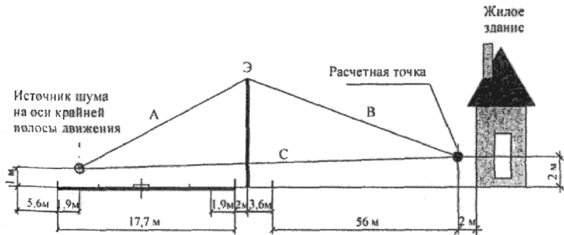
Рис. 4. Расчетная схема оценки эффективности шумозащитного экрана
