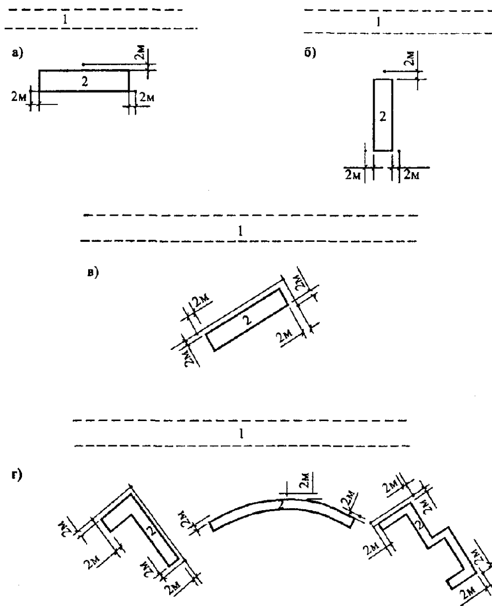
Рис. 4.3. Выбор расчетных точек около здания:
